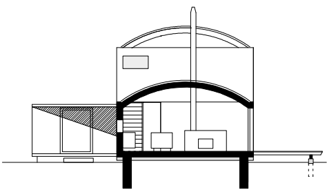
SCHNITT A-A
